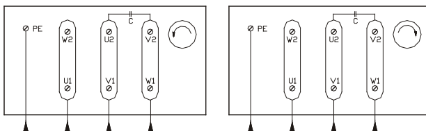
Rys. 4. Schemat podłączenia wentylatorów WDCH z silnikiem jednofazowym z regulatorem obrotów TR
