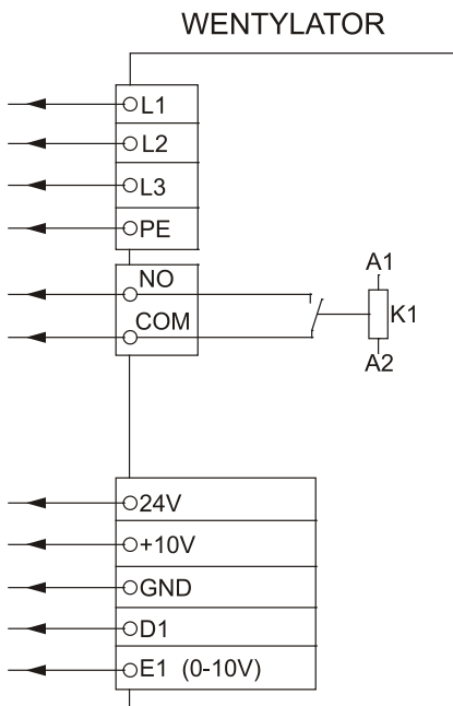
Rys. 12 Schemat podłączenia wentylatora centrali DAWGo...[-1, -2]
