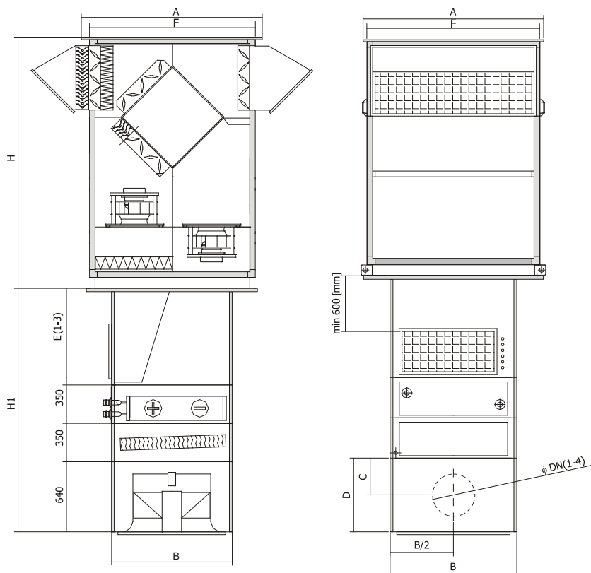
Rys. 2 Podstawowe wymiary aparatu
