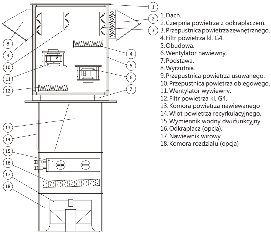
Rys. 1 Budowa aparatu
